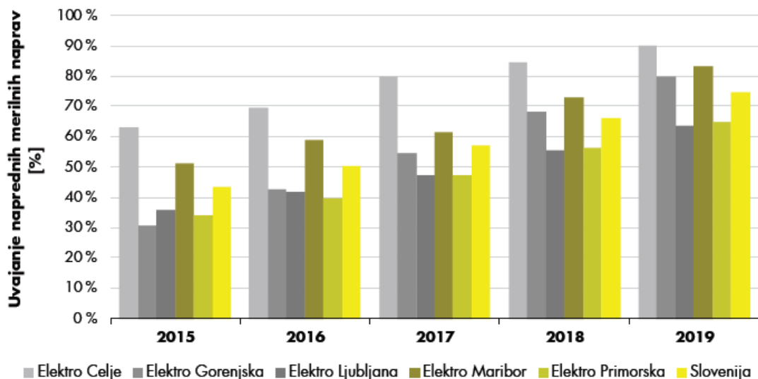
SLIKA 40: TREND UVAJANJA NAPREDNIH MERILNIH NAPRAV V OBDOBJU 2015–2019
