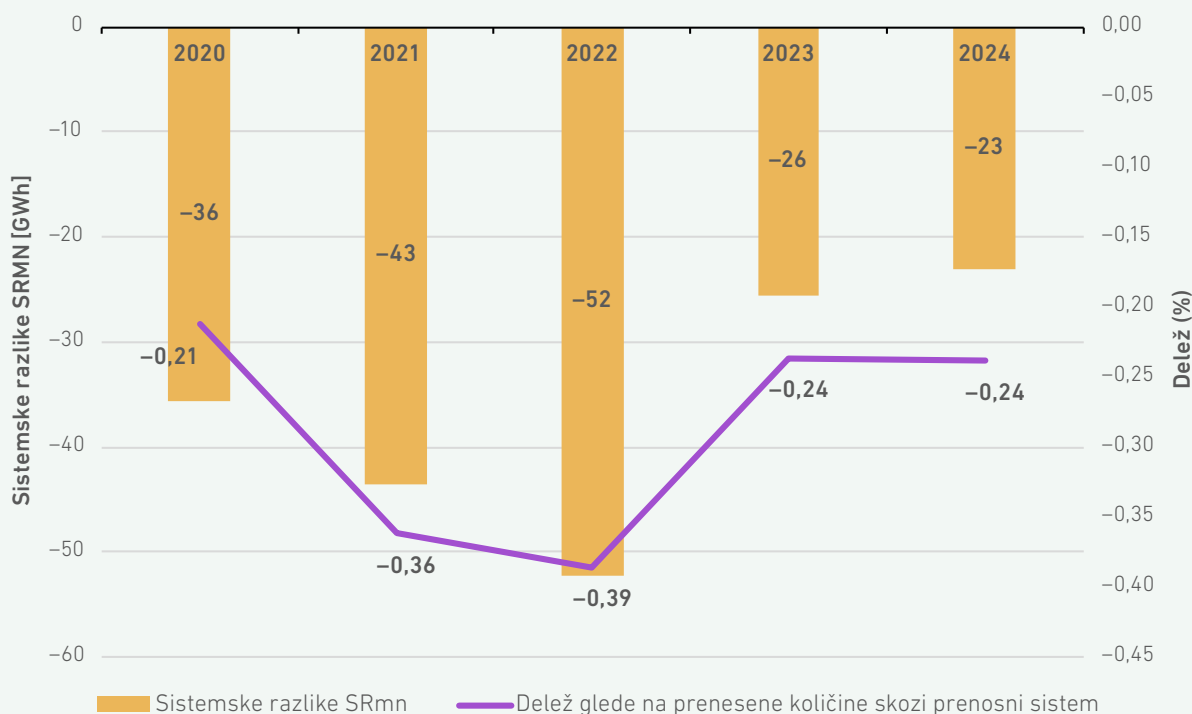
SLIKA 191: SISTEMSKE RAZLIKE SR_{MN} IN DELEŽ GLEDE NA PRENESENE KOLIČINE SKOZI PRENOSNI SISTEM V OBDOBJU 2020–2024
