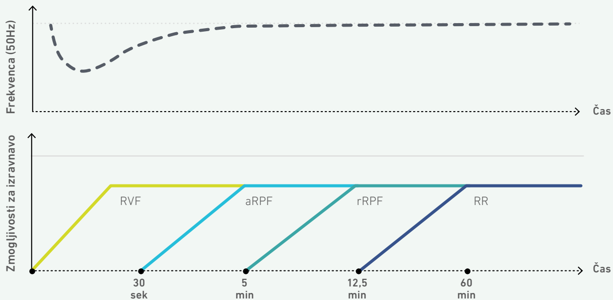
SLIKA 31: PRIMER POSTOPKOV AKTIVACIJ REZERV V PRIMERU POMANJKANJA ZADOSTNIH PROIZVODNIH ZMOGLJIVOSTI
