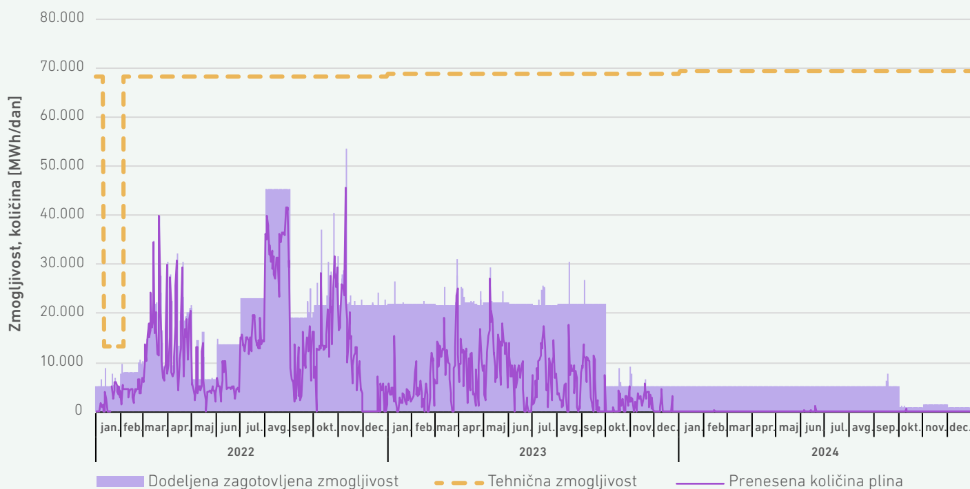
SLIKA 213: DINAMIKA DNEVNO PRENESENIH KOLIČIN PLINA, TEHNIČNA ZMOGLJIVOST IN DODELJENA ZAGOTOVLJENA ZMOGLJIVOST NA IZSTOPNI TOČKI ROGATEC V OBDOBJU 2022–2024
