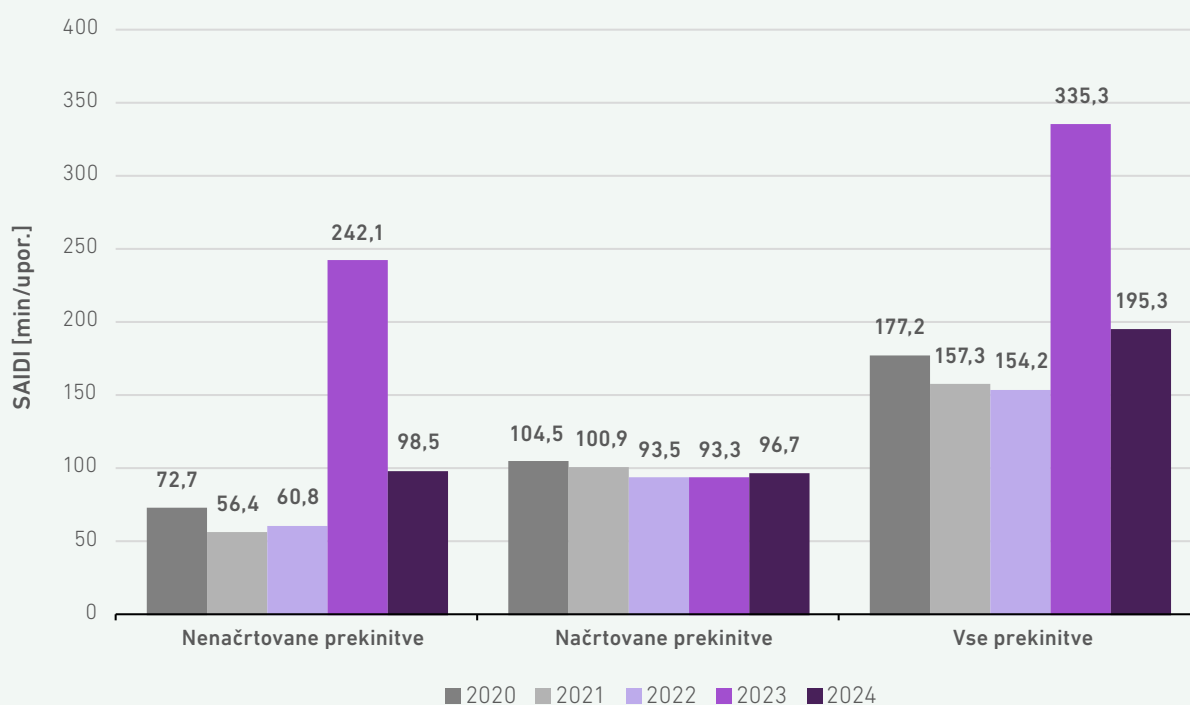
SLIKA 40: PARAMETER SAIDI ZA VSE DOLGOTRAJNE PREKINITVE, LOČENE PO VZROKIH V OBDOBJU 2020–2024
