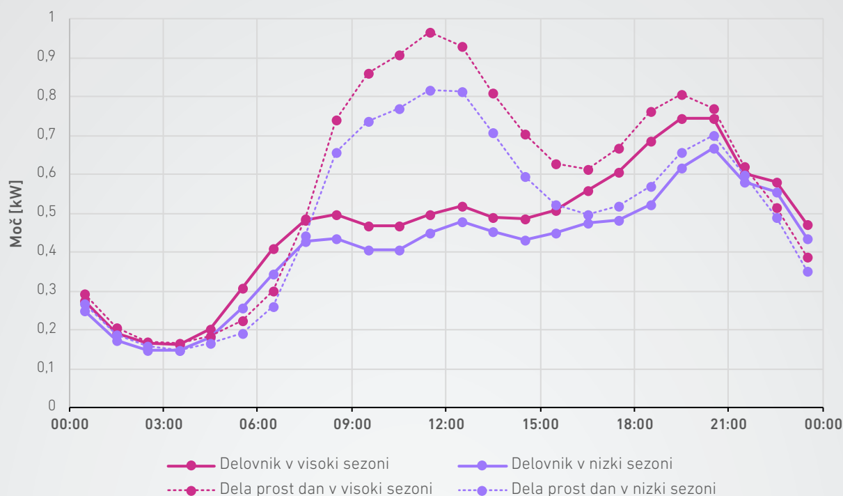
SLIKA 130: SINTETIČNI PROFIL NAVIDEZNEGA GOSPODINJSKEGA ODJEMALCA
