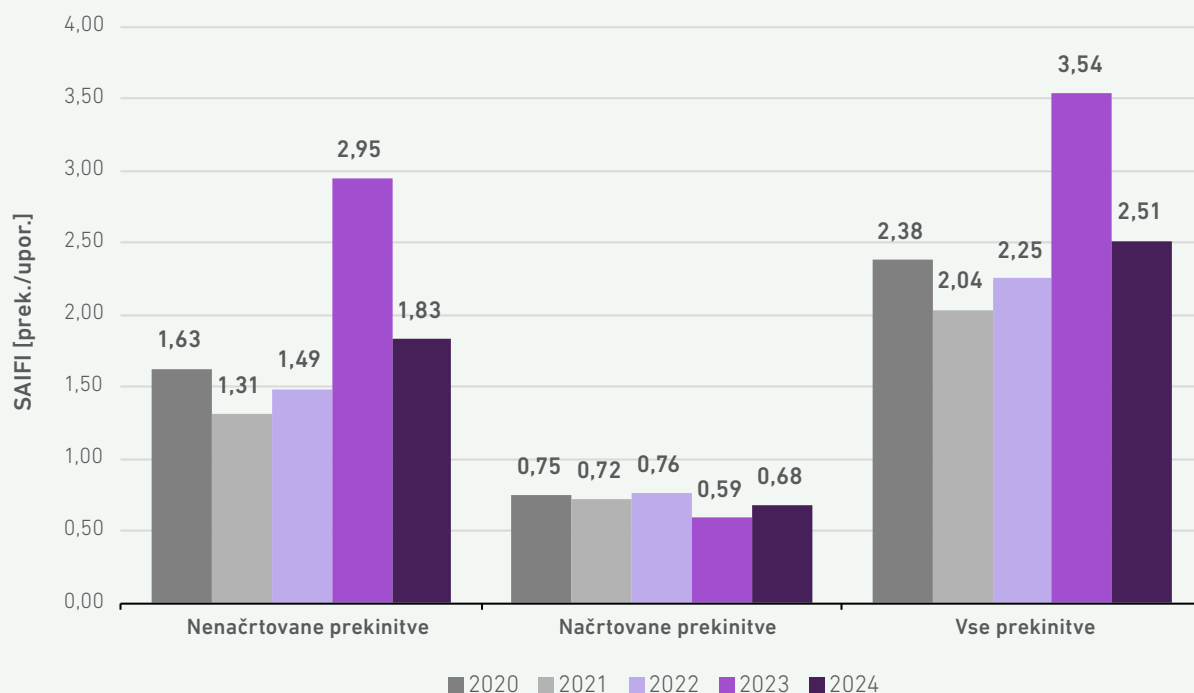
SLIKA 41: PARAMETER SAIFI ZA VSE DOLGOTRAJNE PREKINITVE, LOČENE PO VZROKIH V OBDOBJU 2020–2024
