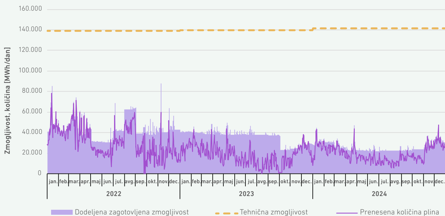
SLIKA 209: DINAMIKA DNEVNO PRENEŠENIH KOLIČIN PLINA, TEHNIČNA ZMOGLJIVOST IN DODELJENA ZAGOTOVLJENA ZMOGLJIVOST NA VSTOPNI TOČKI CERŠAK V OBDOBJU 2022–2024
