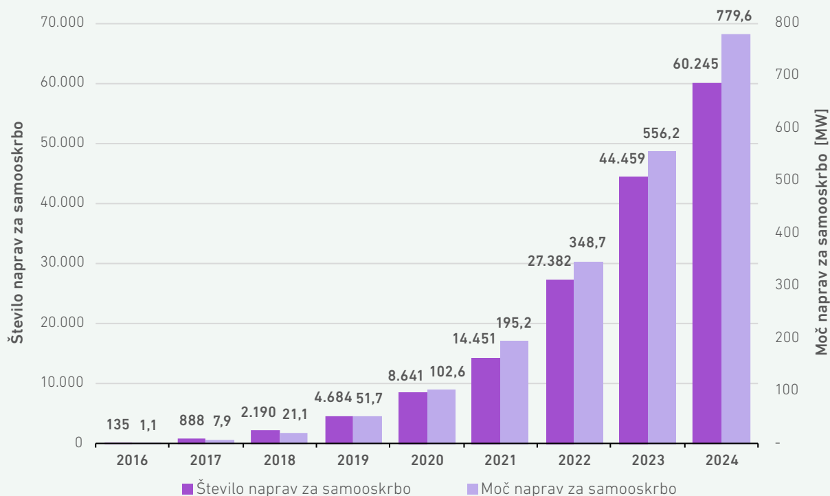
SLIKA 23: ŠTEVILO IN PRIKLJUČNA MOČ NAPRAV ZA SAMOOSKRBO V OBDOBJU 2016–2024
