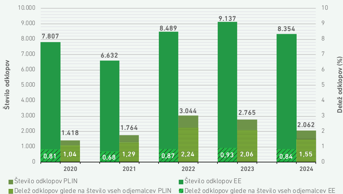
SLIKA 246: PRIMERJAVA ŠTEVILA ODKLOPOV KONČNIH ODJEMALCEV
