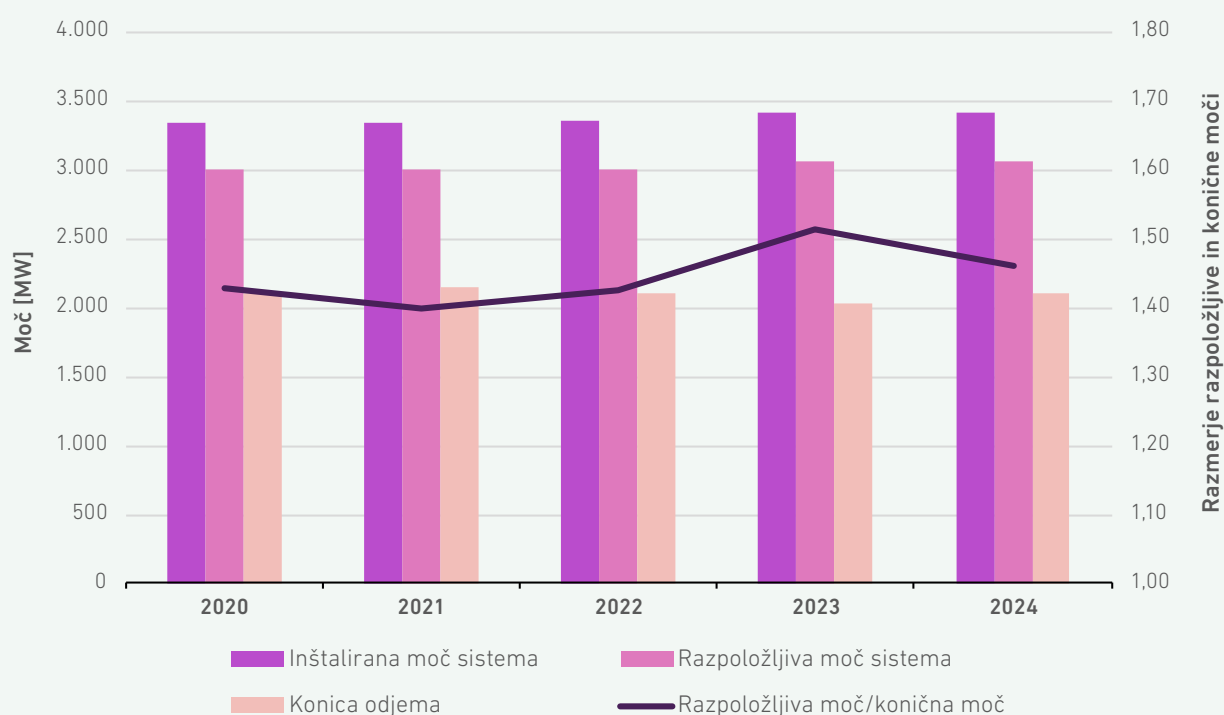
SLIKA 168: INŠTALIRANE MOČI NA PRAGU PROIZVODNIH OBJEKTOV, RAZPOLOŽLJIVE MOČI ZA SLOVENSKI TRG IN KONIČNA MOČ ODJEMA TER RAZMERJE RAZPOLOŽLJIVE IN KONIČNE MOČI NA PRENOSNEM SISTEMU V OBDOBJU 2020–2024
