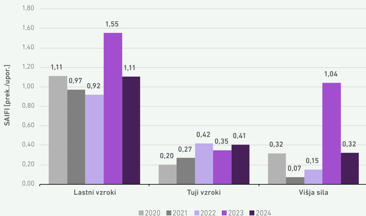
SLIKA 38: PARAMETER SAIFI ZA NENAČRTOVANE DOLGOTRAJNE PREKINITVE, LOČENE PO VZROKIH V OBDOBJU 2020–2024
