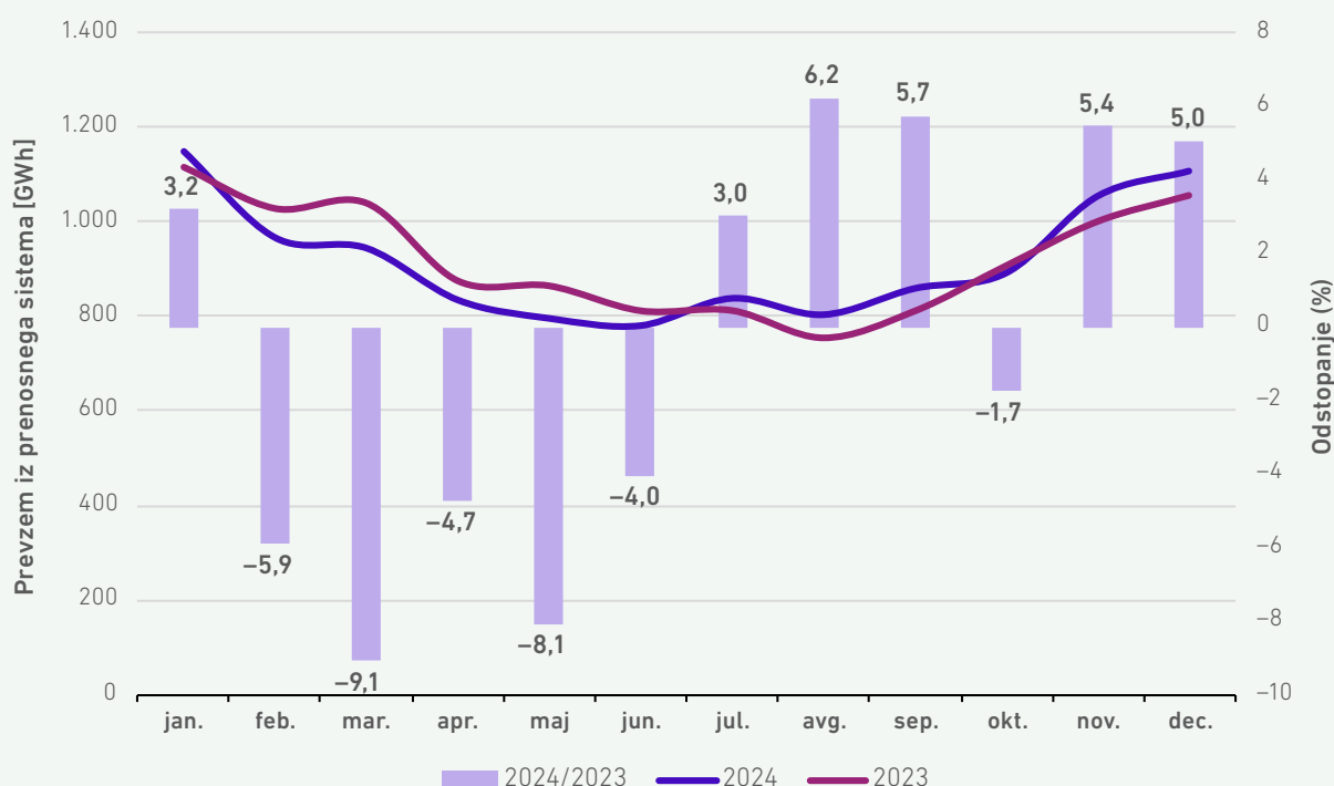
SLIKA 4: MESEČNI PREVZEM ELEKTRIČNE ENERGIJE IZ PRENOSNEGA SISTEMA V LETIH 2023 IN 2024 Z MESEČNIM ODPSTOPANJEM
