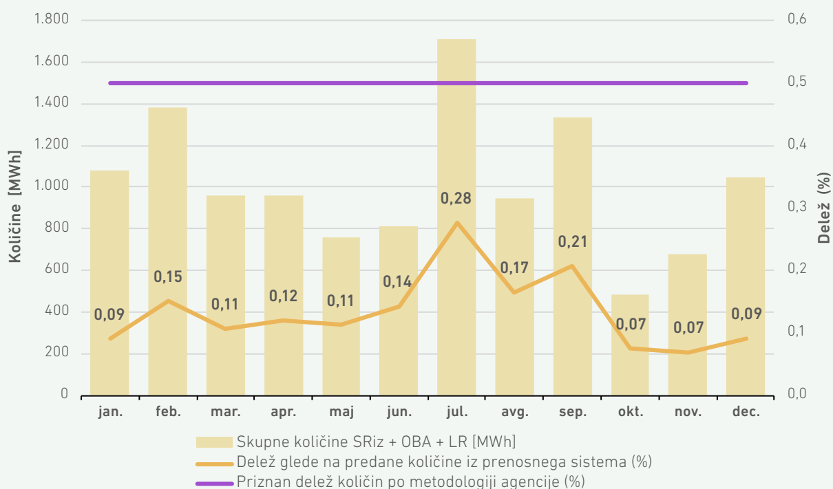
SLIKA 192: MESEČNO GIBANJE VSOTE SISTEMSKIH RAZLIK SR IZ , KOLIČIN ZA LASTNO RABO IN KOLIČIN ZA NAMEN OBRAČUNA PO OBA V LETU 2024
