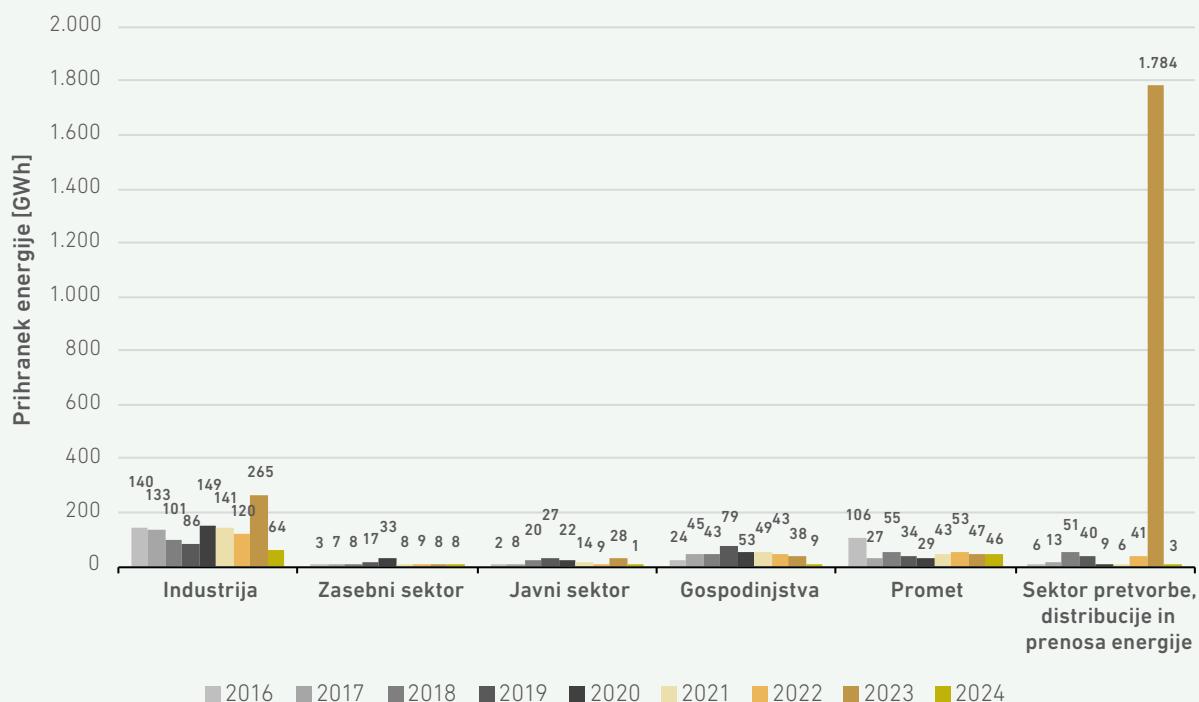
SLIKA 260: DOSEŽENI PRIHRANKI ENERGIJE PO SEKTORJIH V OBDOBJU 2016–2024
