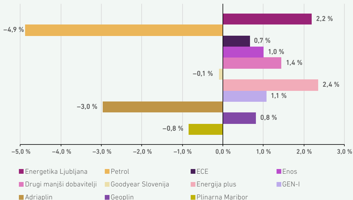
SLIKA 234: SPREMEMBE TRŽNIH DELEŽEV NA TRGU ZA KONČNE ODJEMALCE V LETU 2024 GLEDE NA LETO 2023 149
