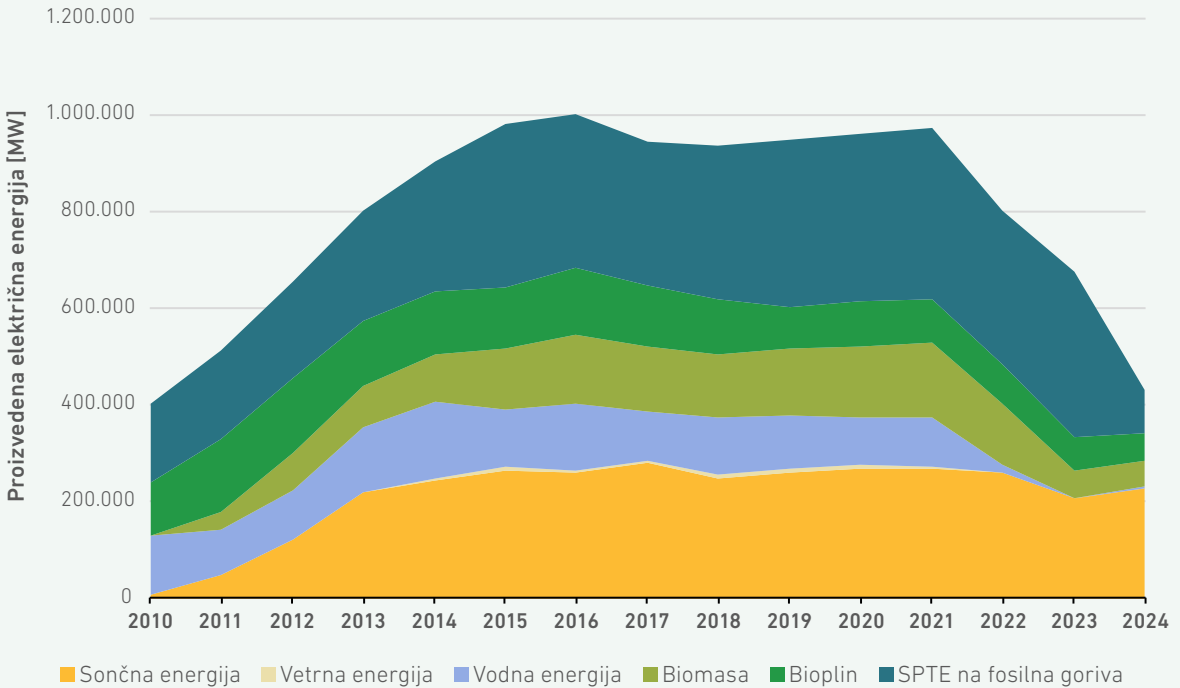
SLIKA 21: PROIZVEDENA ELEKTRIČNA ENERGIJA V OBDOBJU OD 2010–2024, ZA KATERO SO BILE PROIZVAJALCEM ELEKTRIČNE ENERGIJE IZPLAČANE PODPORE
