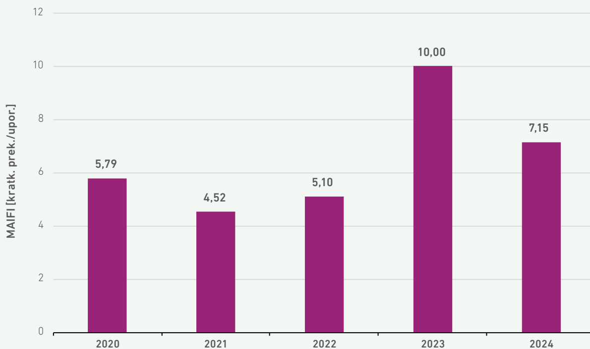
SLIKA 39: PARAMETER MAIFI V OBDOBJU 2020–2024
