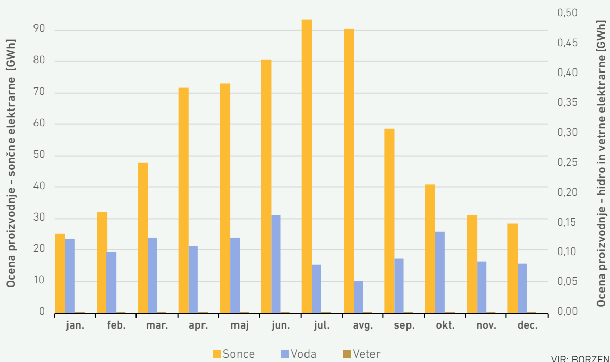
SLIKA 25: OCENA PROIZVODNJE NAPRAV ZA SAMOOSKRBO V LETU 2024 PO MESECIH IN TEHNOLOGIJAH
