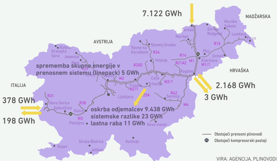
SLIKA 171: PRENOSNI SISTEM PLINA IN PRENESENE KOLIČINE PLINA NA VSTOPNIH IN IZSTOPNIH TOČKAH V 2024
