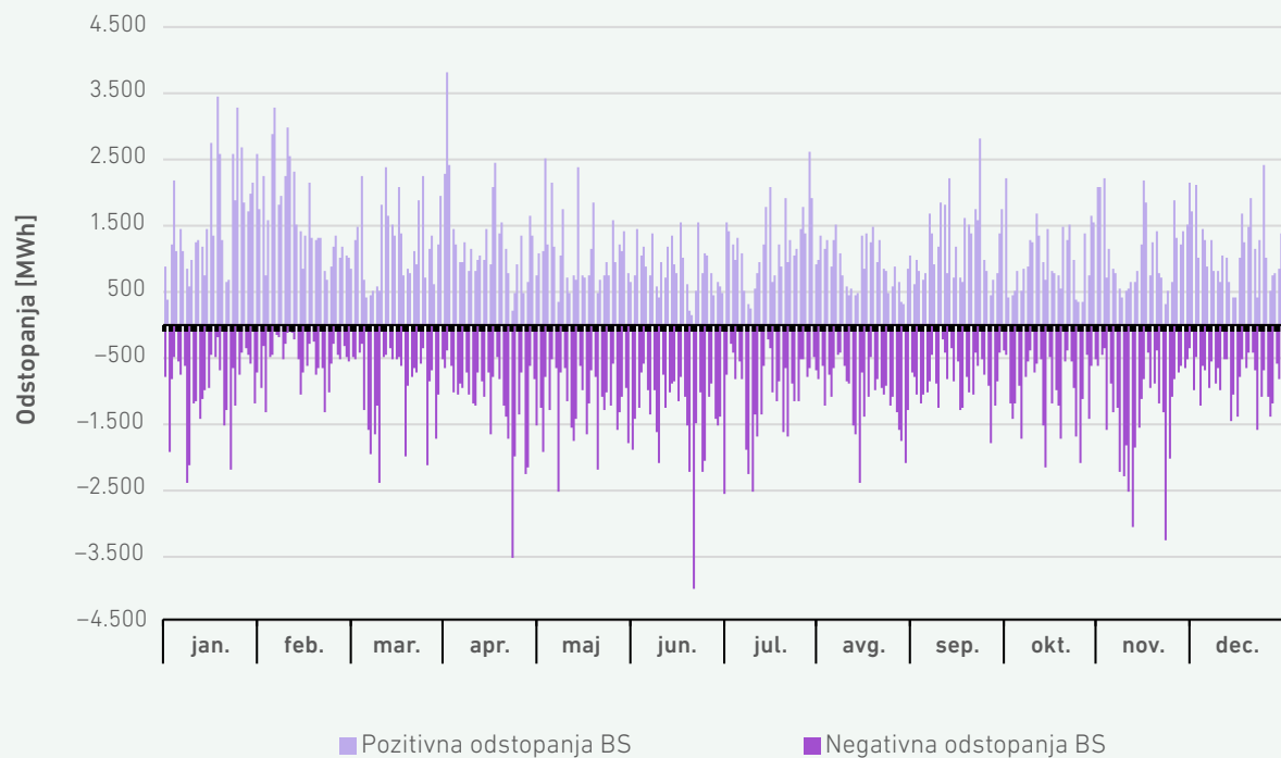
SLIKA 35: DNEVNA ODSTOPANJA OD NAPOVEDI PORABE V SLOVENSKEM OMREŽJU V LETU 2024
