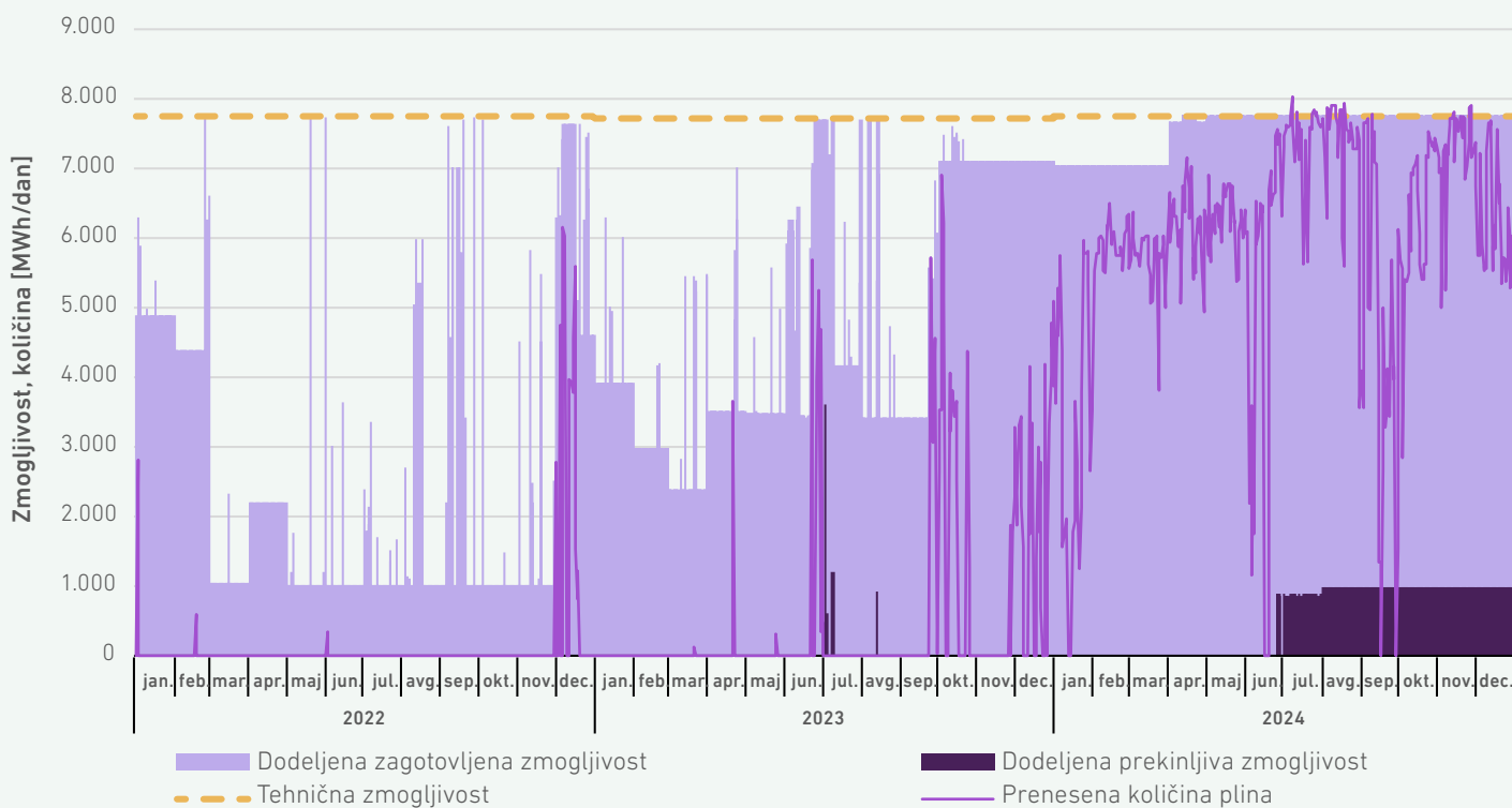
SLIKA 212: DINAMIKA DNEVNO PRENESENH KOLIČIN PLINA, TEHNIČNA ZMOGLJIVOST, DODELJENA ZAGOTOVLJENA IN PREKINLJIVA ZMOGLJIVOST NA VSTOPNI TOČKI ROGATEC V OBDOBJU 2022–2024
