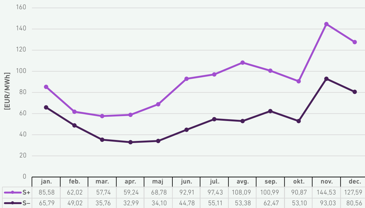
SLIKA 36: POVPREČNE MESEČNE VREDNOSTI STROŠKOV REGULACIJE (S+ IN S-) V LETU 2024
