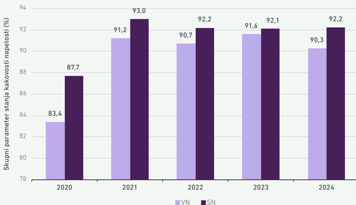
SLIKA 42: SKUPNI PARAMETER STANJA KAKOVOSTI NAPETOSTI ZA POSAMEZEN NAPETOSTNI NIVO V DISTRIBUCIJSKEM SISTEMU V OBDOBJU 2020–2024
