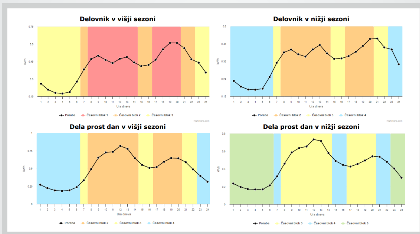
SLIKA 135: SINTETIČNI PROFIL NAVIDEZNEGA GOSPODINJSKEGA ODJEMALCA Z VAROVALKO 3 X 25 A S PORABO MED 2,5 MWh IN 5 MWh (VIZUALIZIRANI SO VELJAVNI OMREŽNINSKI ČASOVNI BLOKI)
