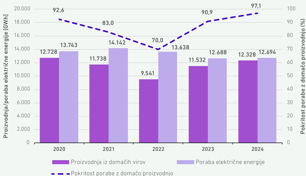
SLIKA 13: PORABA, PROIZVODNJA IN POKRITOST PORABE Z DOMAČO PROIZVODNJO V OBDOBJU 2020–2024
