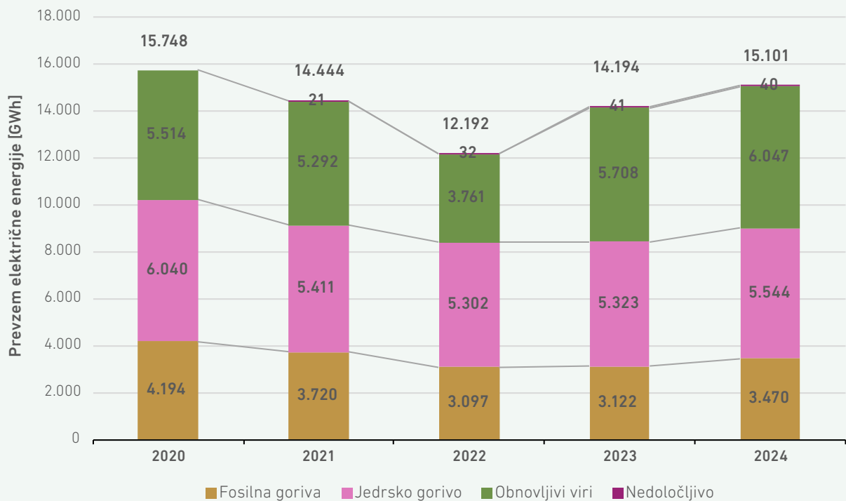
SLIKA 8: PREVZEM ELEKTRIČNE ENERGIJE IZ PROIZVODNIH ENOT V PRENOSNI IN DISTRIBUCIJSKI SISTEM V OBDOBJU 2020–2024
