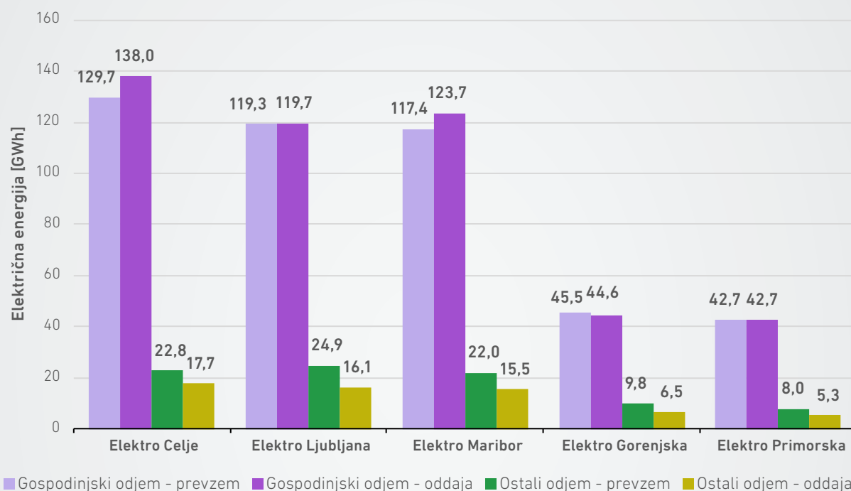
SLIKA 27: KOLIČINA PREVZETE IN ODDANE ELEKTRIČNE ENERGIJE SAMOOSKRBNIH ODJEMALCEV PO OBMOČJIH DISTRIBUCIJSKEGA SISTEMA V LETU 2024
