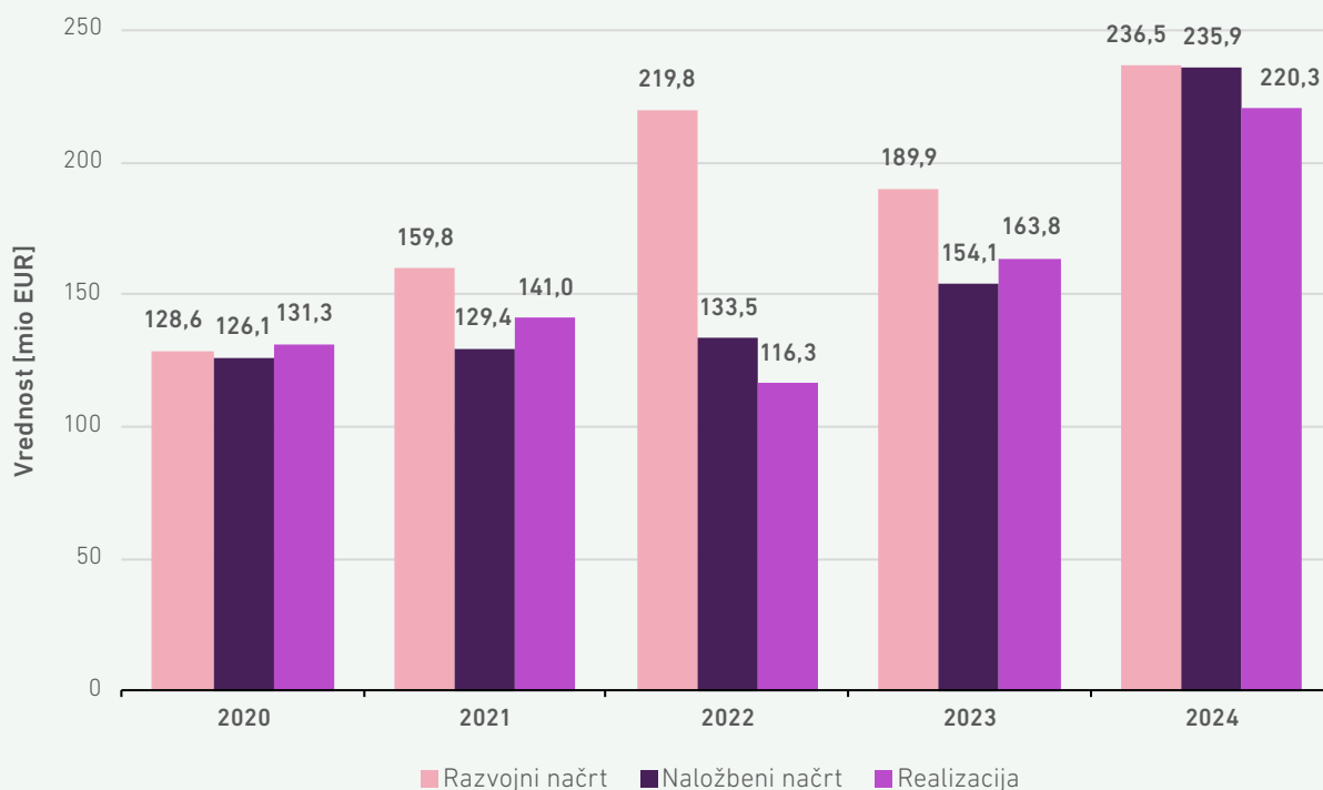
SLIKA 46: PRIMERJAVA VREDNOSTI V RAZVOJNIH IN NALOŽBENIH NAČRTIH ZA DISTRIBUCIJSKI SISTEM ELEKTRIČNE ENERGIJE TER REALIZACIJA
