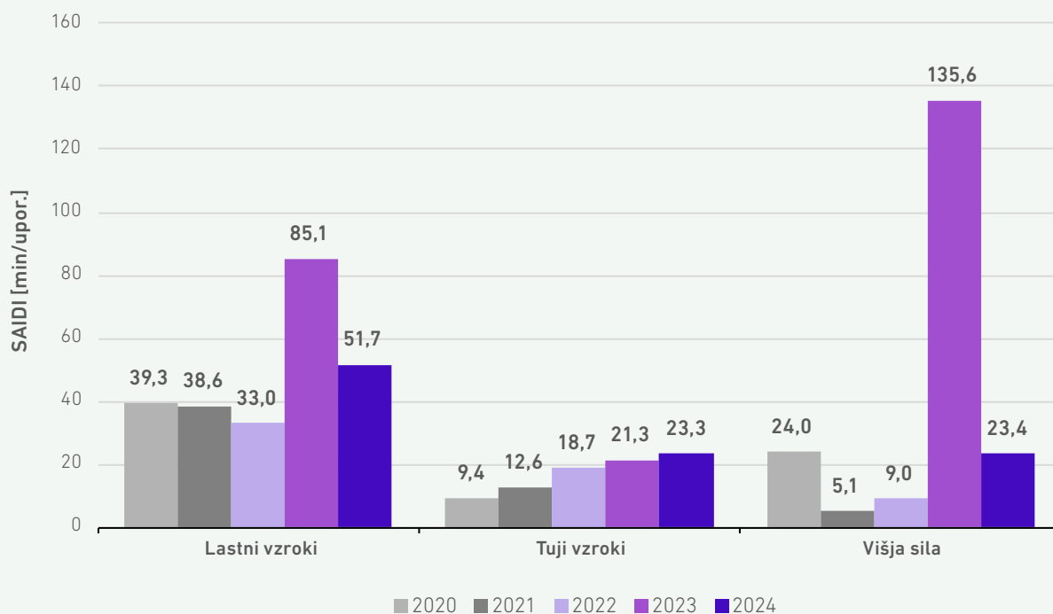
SLIKA 37: PARAMETER SAIDI ZA NENAČRTOVANE DOLGOTRAJNE PREKINITVE, LOČENE PO VZROKIH V OBDOBJU 2020–2024
