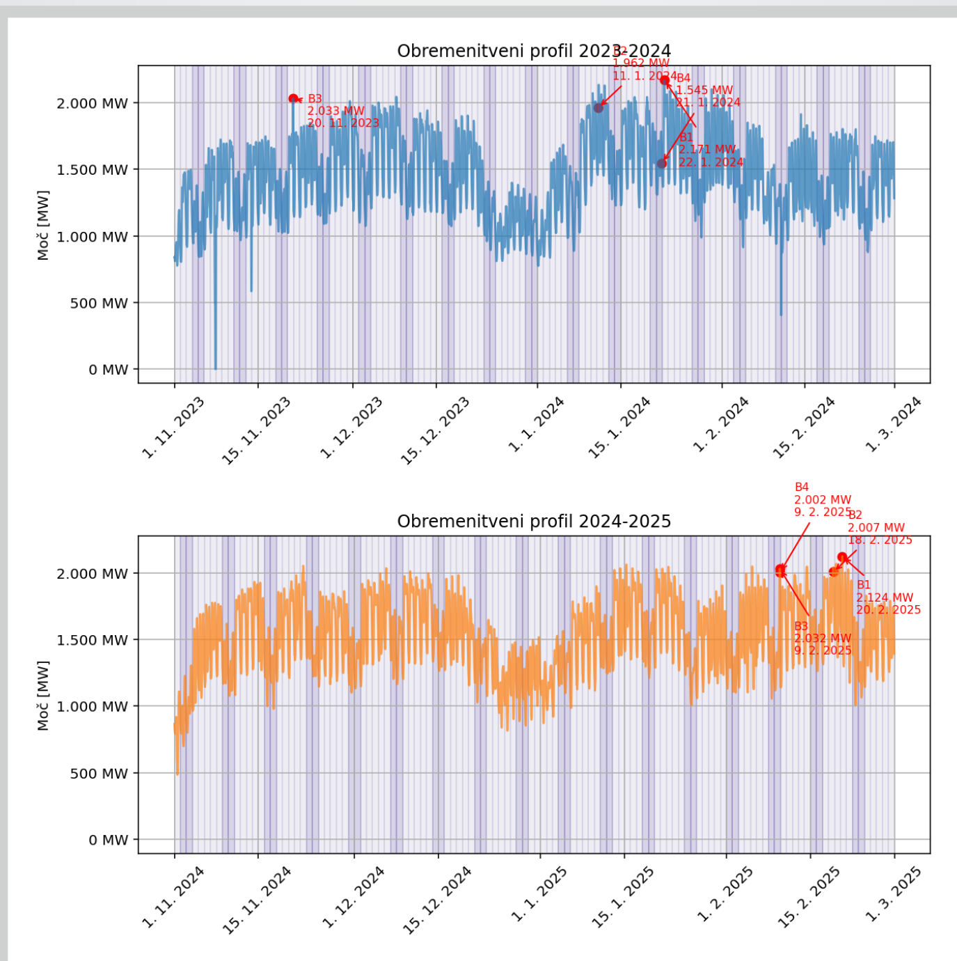
SLIKA 75: ANALIZA SISTEMSKIH KONIČNIH OBREMENITEV V OBDOBJIH ZADNJIH VIŠJIH SEZON
