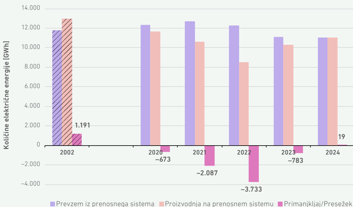
SLIKA 167: PREVZEM IN PROIZVODNJA ELEKTRIČNE ENERGIJE V SLOVENIJI NA PRENOSNEM SISTEMU BREZ UPOŠTEVANJA IZGUB V OBDOBJU 2020–2024 IN PRIMERJAVA Z LETOM 2002
