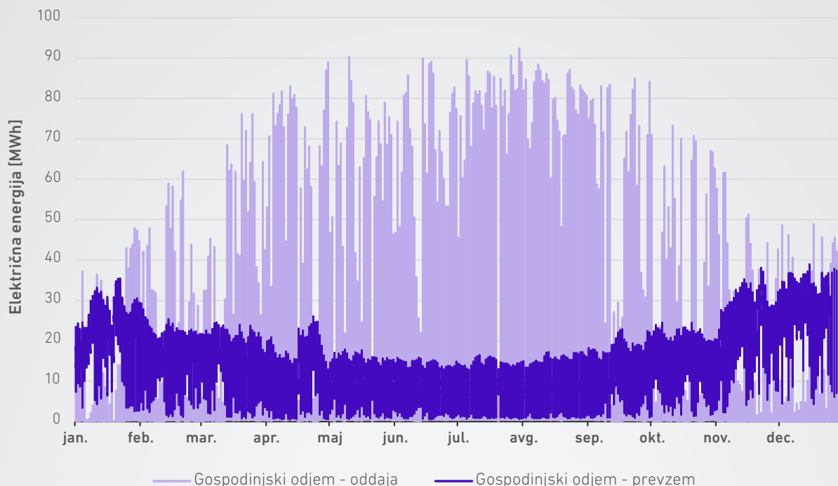
SLIKA 28: AGREGIRAN PROFIL PROIZVODNJE IN PORABE VSEH SAMOOSKRBNIH GOSPODINJSKIH ODJEMALCEV V LETU 2024
