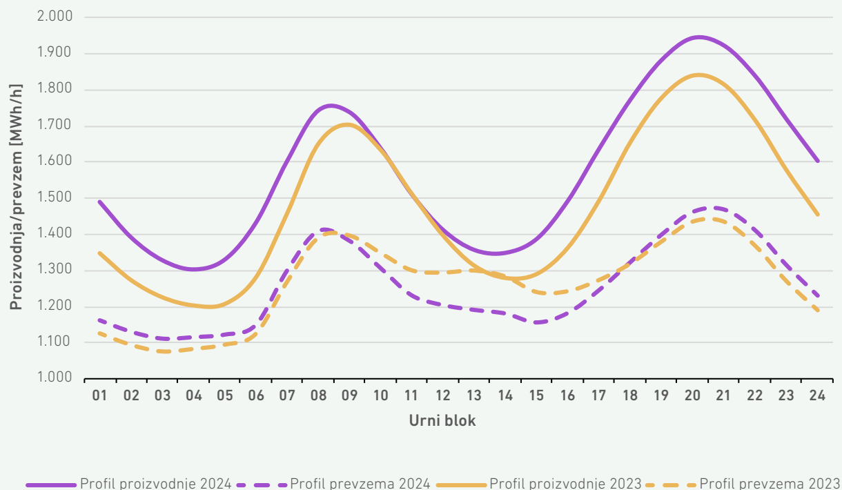
SLIKA 7: POVPREČNI DNEVNI PROFIL PROIZVODNJE IN PREVZEMA ELEKTRIČNE ENERGIJE IZ PRENOSNEGA SISTEMA V LETIH 2023 IN 2024
