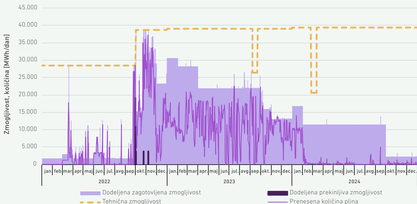
SLIKA 210: DINAMIKA DNEVNO PRENESENH KOLIČIN PLINA, TEHNIČNA ZMOGLJIVOST, DODELJENA ZAGOTOVLJENA IN PREKINLJIVA ZMOGLJIVOST NA VSTOPNI TOČKI ŠEMPETER V OBDOBJU 2022–2024
