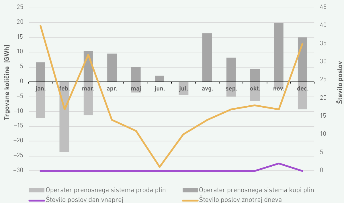
SLIKA 224: TRGOVANJE NA TRGOVALNI PLATFORMI V LETU 2024
