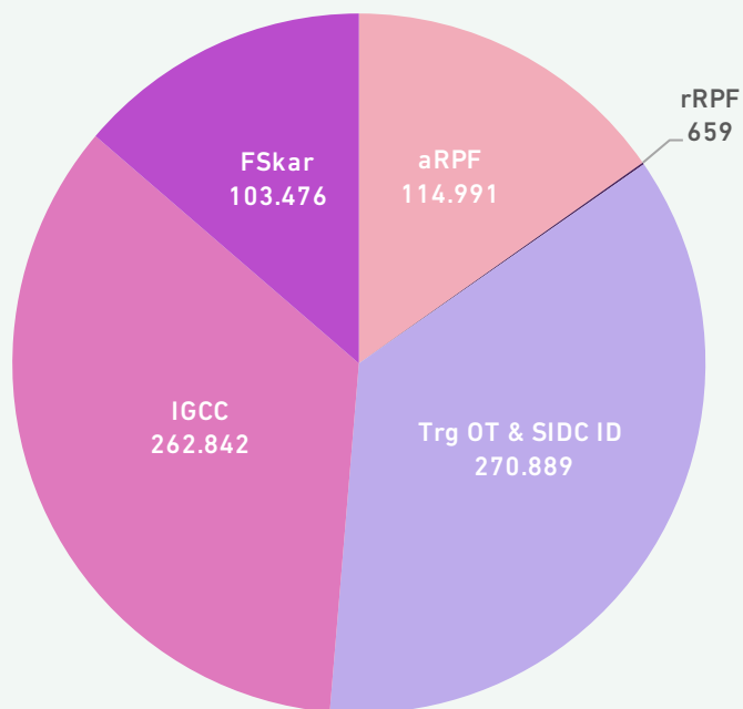
SLIKA 107: ABSOLUTNE VREDNOSTI ANGAŽIRANIH KOLIČIN IZRAVNALNE ENERGIJE V MWh
