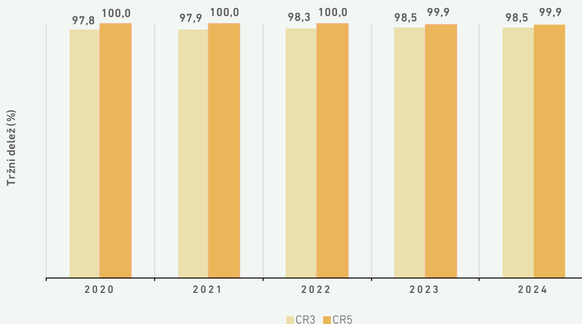
SLIKA 220: KONCENTRACIJA VELEPRODAJNEGA TRGA S PLINOM
