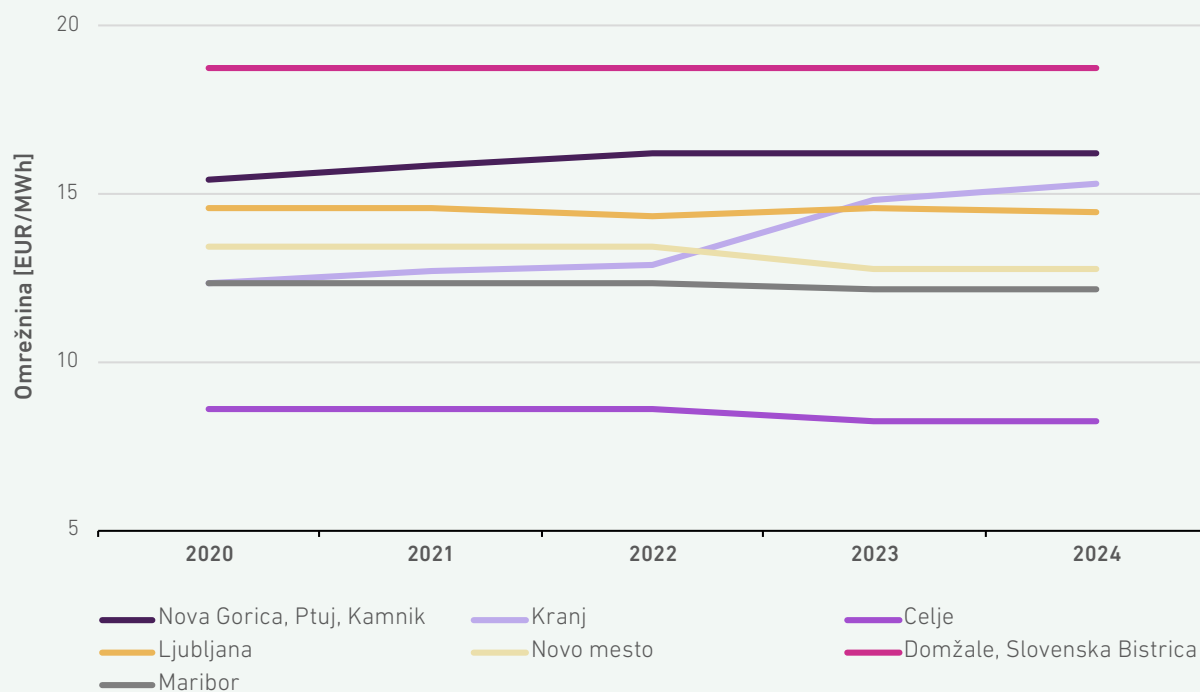
SLIKA 204: GIBANJE OMREŽNINE ZA DISTRIBUCIJO ZA SREDNJE VELIKE GOSPODINJSKE ODJEMALCE – D2 (32 MWh) V OBDOBJU 2020–2024
