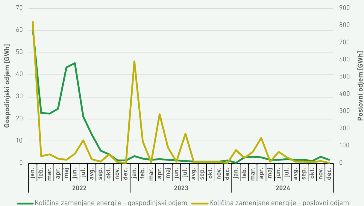
SLIKA 146: KOLIČINE ZAMENJANE ENERGIJE GLEDE NA TIP ODJEMA
