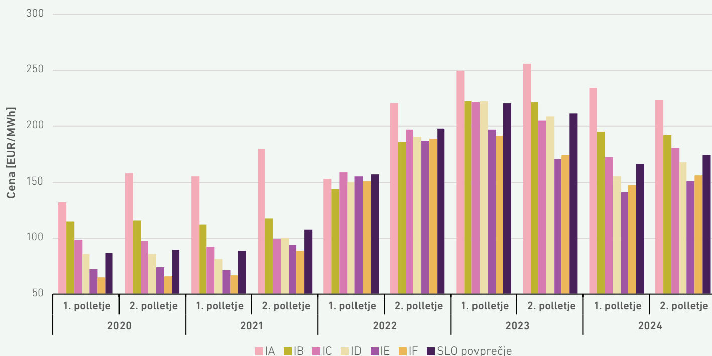
SLIKA 116: GIBANJE KONČNE CENE OSKRBE Z ELEKTRIČNO ENERGIJO V SLOVENIJI ZA ZNAČILNE POSLOVNE ODJEMALCE V OBDOBJU 2020–2024
