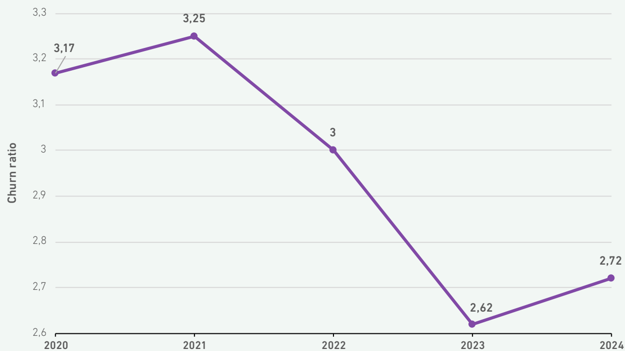
SLIKA 109: TREND GIBANJA INDEKSA »CHURN RATIO« PO LETIH V OBDOBJU 2020–2024
