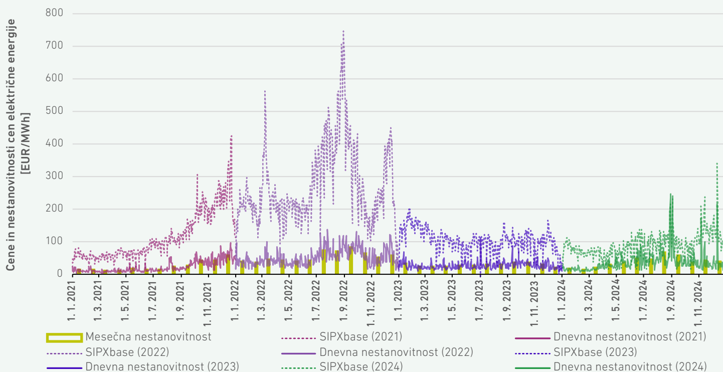
SLIKA 126: RAZVOJ CEN TER NESTANOVITNOSTI CEN NA SLOVENSKI ENERGETSKI BORZI
