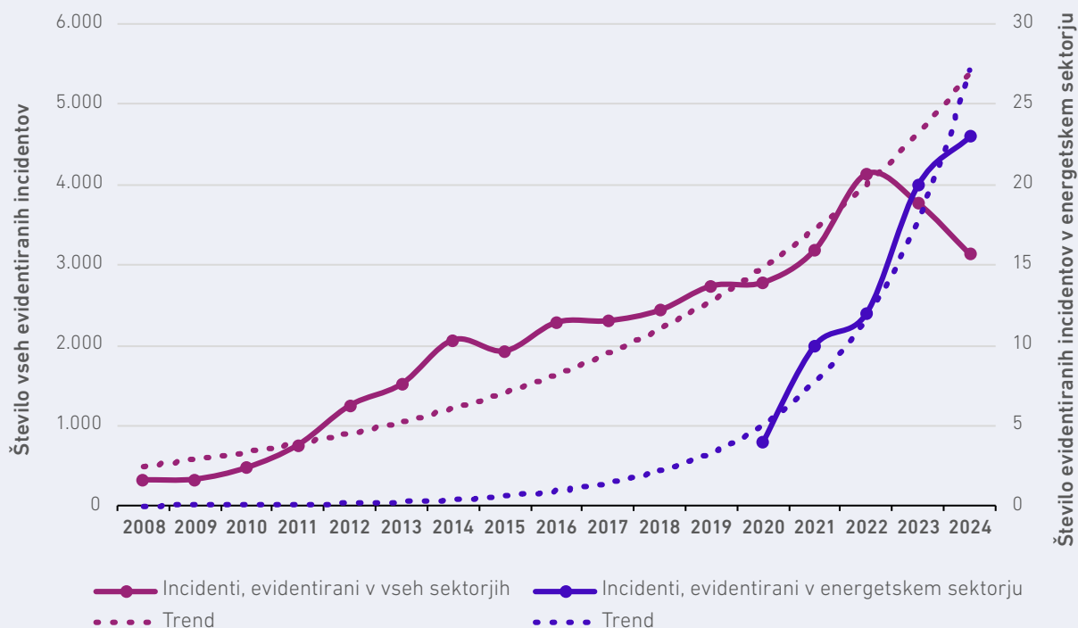
SLIKA 66: DOLGOROČNA PROJEKCIJA (EKSPONENTNA OZ. »WORST-CASE« APROKSIMACIJA) RASTI INCIDENTOV V SEKTORJU
