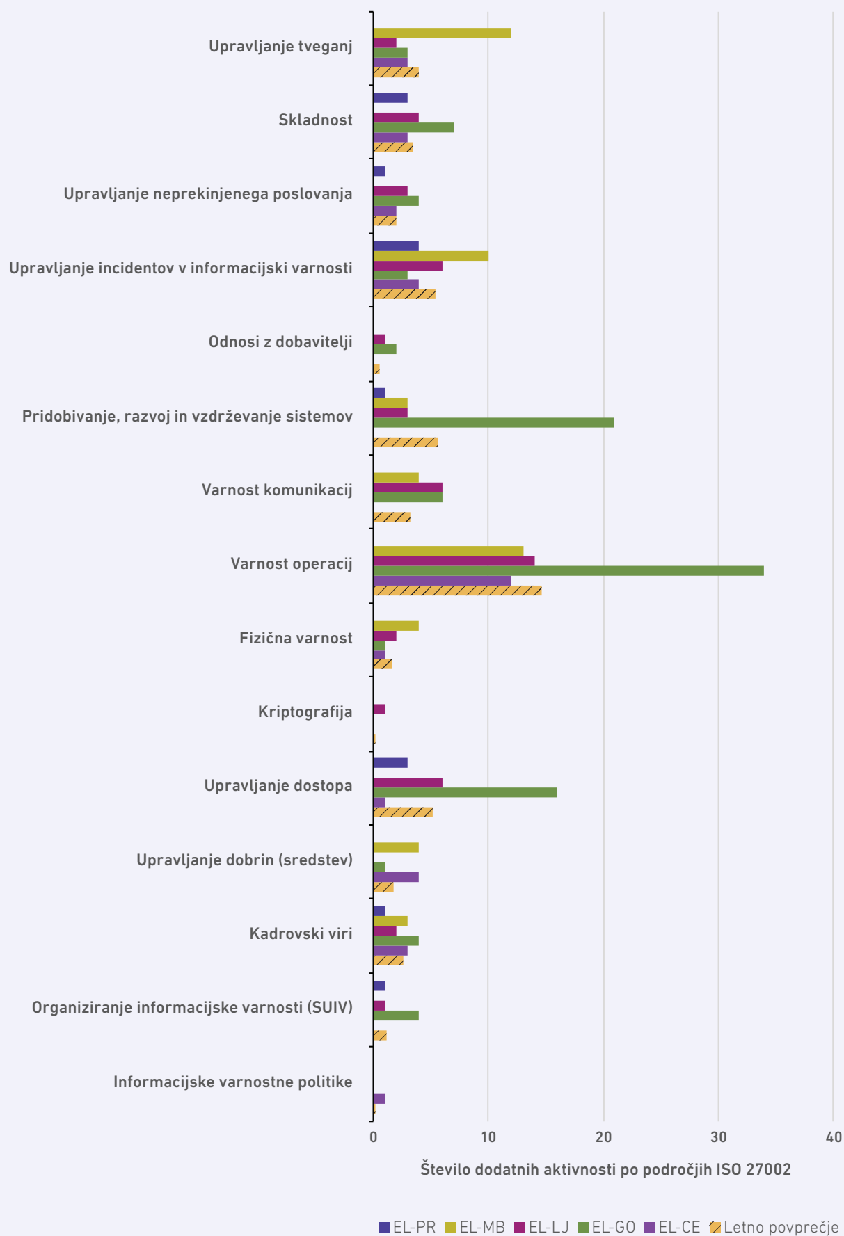
SLIKA 62: PORAZDELITEV OBSEGA AKTIVNOSTI EDP PO PODROČJIH GLEDE NA LETNO POVPREČJE
