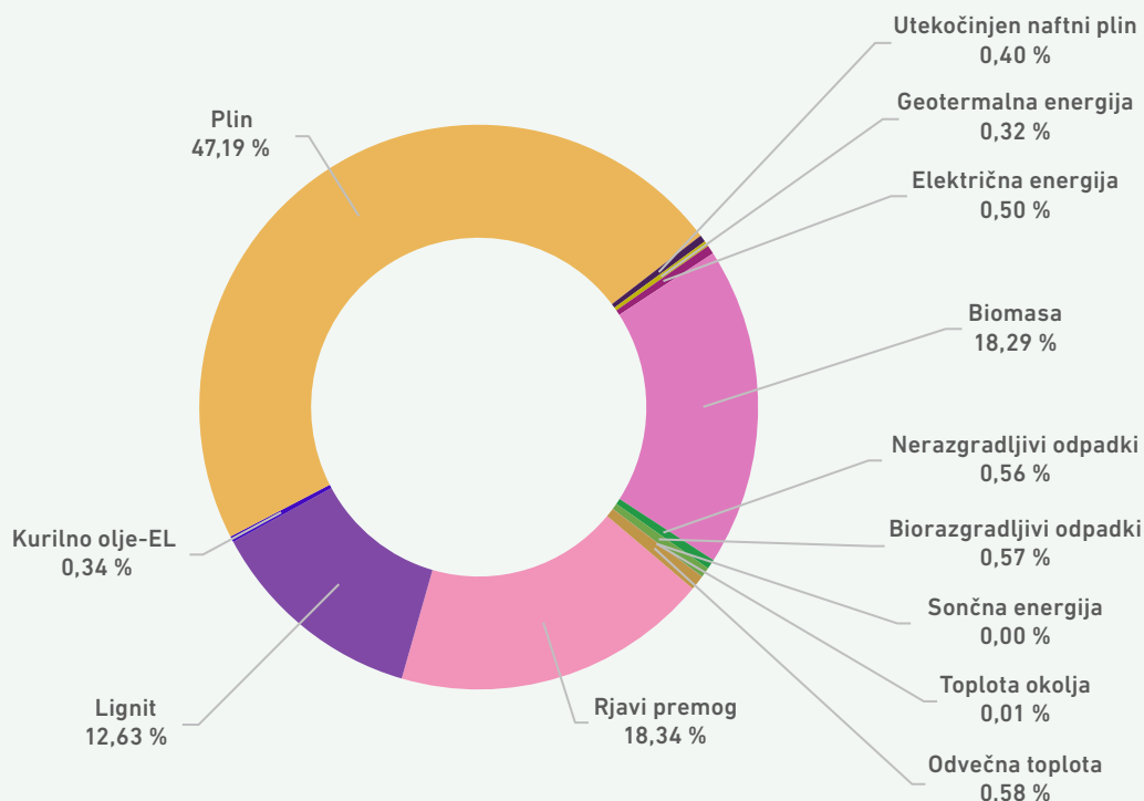
SLIKA 266: STRUKTURA PRIMARNIH ENERGENTOV ZA PROIZVODNJO TOPLOTE
