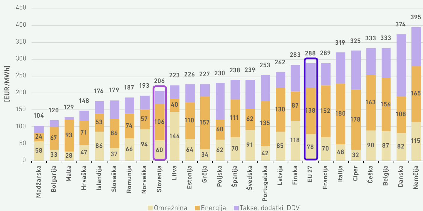
SLIKA 120: PRIMERJAVA DELEŽEV V SKUPNI CENI OSKRBE Z ELEKTRIČNO ENERGIJO ZA ZNAČILNEGA GOSPODINJSKEGA ODJEMALCA V DRŽAVAH EU
