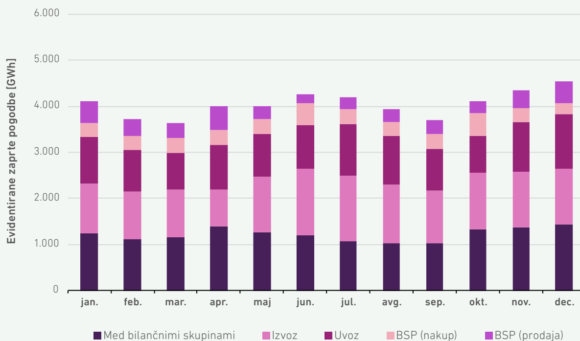
SLIKA 100: KOLIČINE PRODANE OZIROMA KUPLJENE ELEKTRIČNE ENERGIJE PREK ZAPRTIH POGODB
