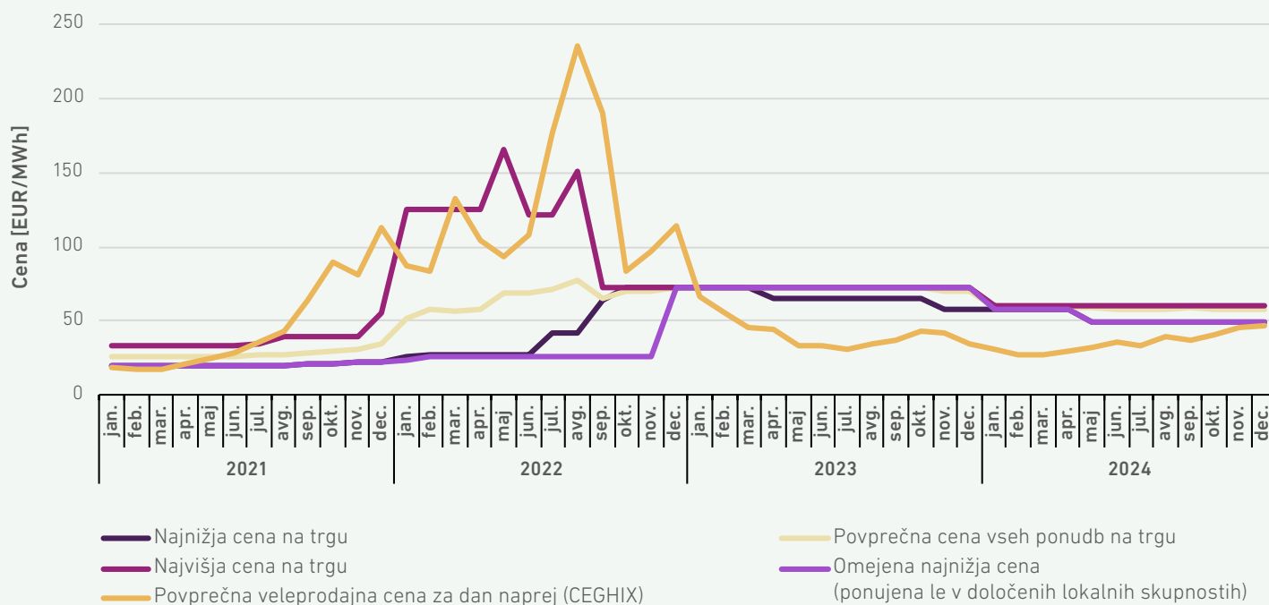
SLIKA 227: MALOPRODAJNI INDEKS CEN IN NEKATERE ZNAČILNE CENE PLINA ZA GOSPODINJSKE ODJEMALCE BREZ OMREŽNINE, DAJATEV IN DDV V OBDOBJU 2021–2024
