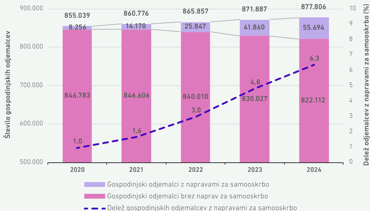
SLIKA 14: ŠTEVILO GOSPODINJSKIH ODJEMALCEV V OBDOBJU 2020–2024
